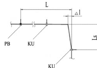
рис. 10: Создание предварительного напряжения в трубопроводе для распределения теплой воды в изгибе трубопроводной линии.
