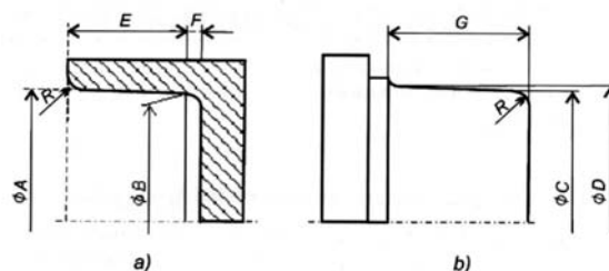
Рис. 29: Полифузионные наконечники, тип А (размеры см. табл. 6).
