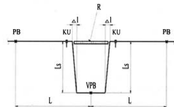
рис. 9: Создание предварительного напряжения в трубопроводе для распределения теплой воды с помощью U — компенсатора.
