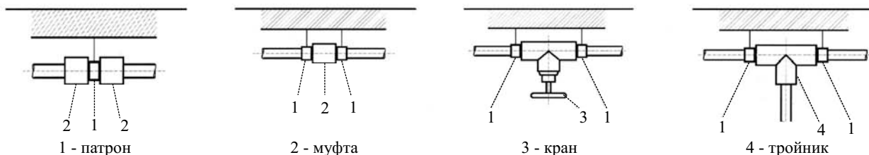
рис. 3: Примеры образования прочных опорных точек с помощью фасонины и патროнов:
