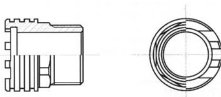
рис. 19. Металлическая резьба, наружная "впрыск".
