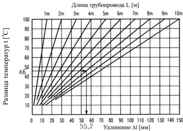
график 1: Удлинение трубопровода \Delta l из полипропилена в зависимости от разницы температур \Delta t транспортируемой среды и длине трубопровода L .
