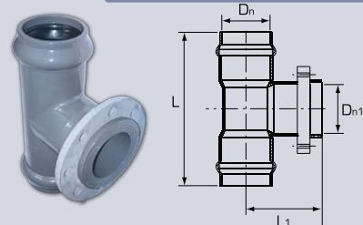
Тройник ПВХ с металлическим фланцем SDR 26. Рабочее давление МОР 1,0 Мпа
