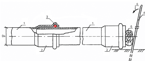
Рис. 1 Раструбное соединение с помощью рычага (1 – ПВХ трубы; 2 – раструб; 3 – резиновое уплотнительное кольцо; 4 – рычаг; 5 – деревянная прокладка; 6 – направление усилия)
